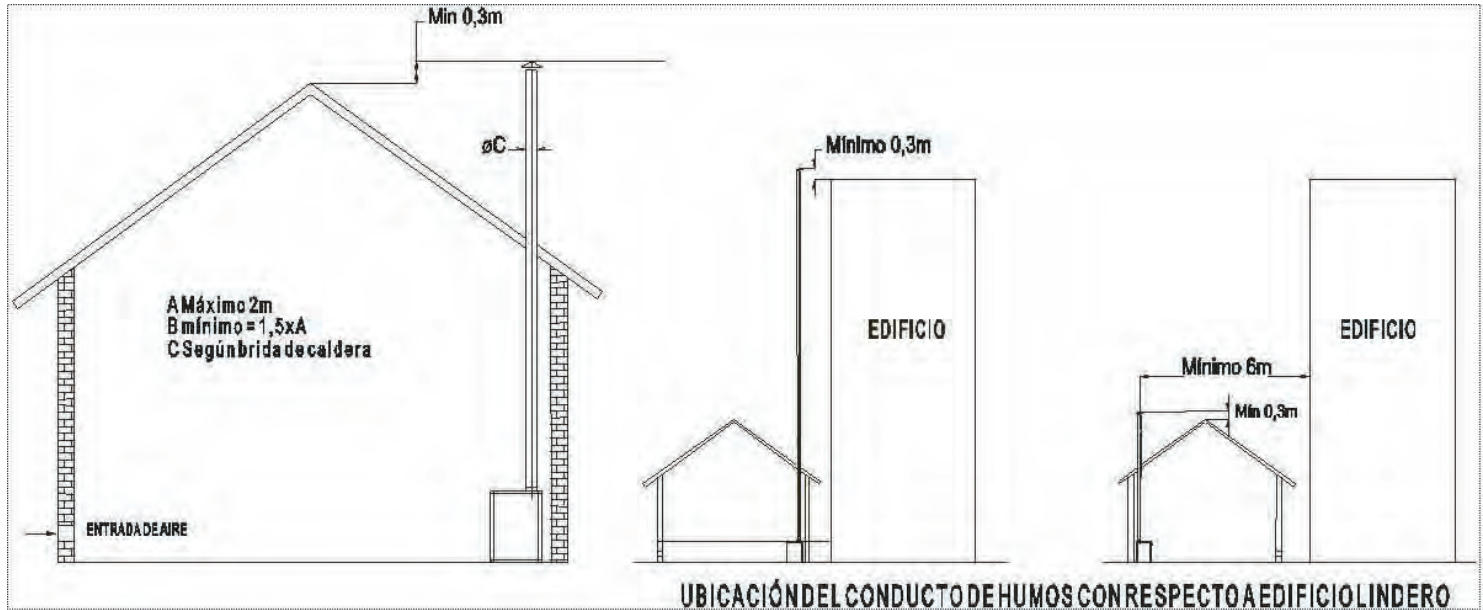
Figura 2: SALIDA DIRECTA
