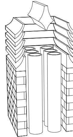
Figura 4: SOMBRERETE MÚLTIPLE
