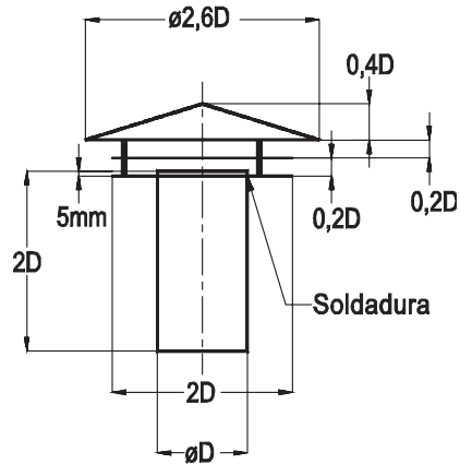
Figura 3: SOMBRERETE INDIVIDUAL
