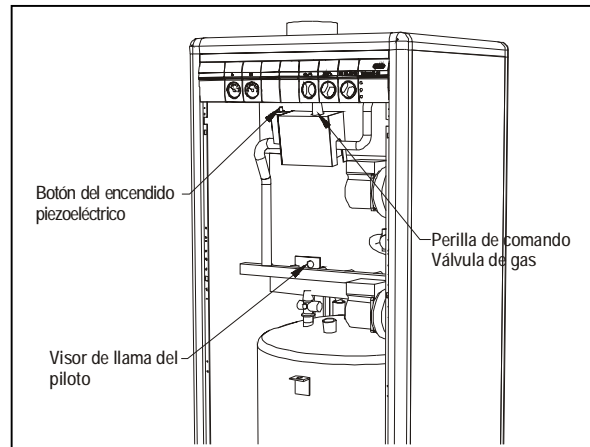
C.- Detalle del pulsador de encendido y válvula de gas
