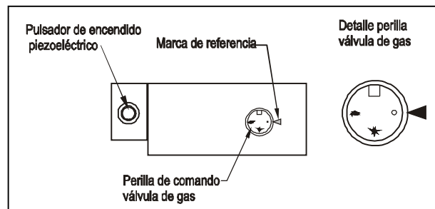
C.- Detalle del pulsador de encendido y válvula de gas
